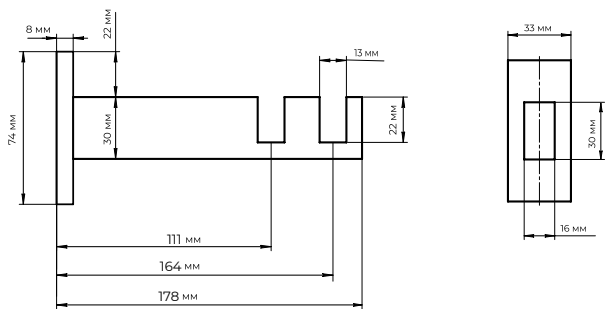
ДЕРЖАТЕЛЬ 2-РЯДНЫЙ 105.910
