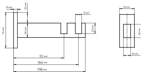
ДЕРЖАТЕЛЬ 2-РЯДНЫЙ 105.904
