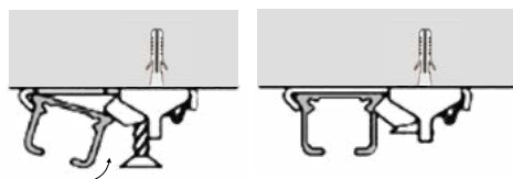
Крепление профиля
