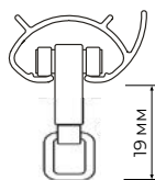
Глайдер роликовый
