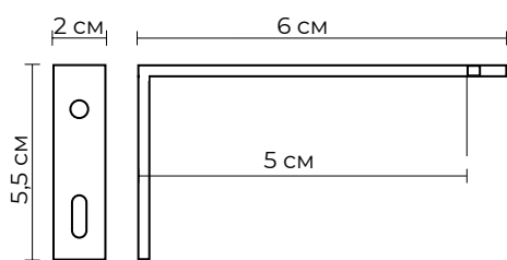
Кронштейн стеновой с крышкой / без крышки 6 см
