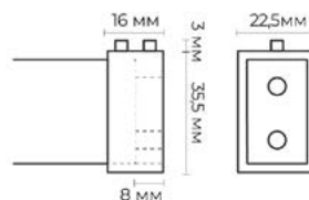
Торцевое крепление для профиля 17x30мм
