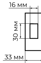
Держатель трехрядный
