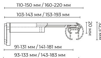
Однорядный телескопический держатель 14-18 см
