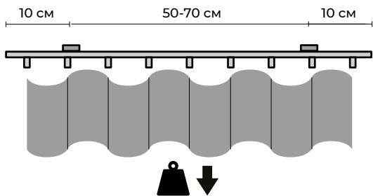
Распределенная нагрузка 15 кг на 1 пог.м карниза
