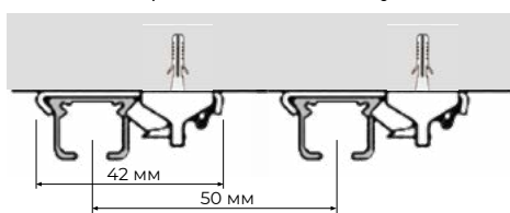
Крепление профиля
