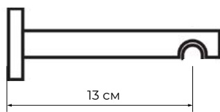
Держатель однорядный
