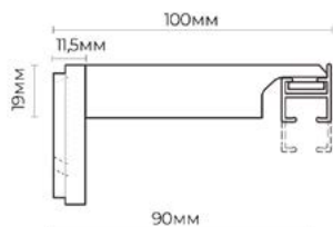
Однорядный держатель 9 см
