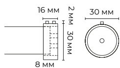
Торцевое крепление для профиля 17x20мм
