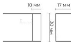
Наконечник Заглушка для профиля 17x30 мм
