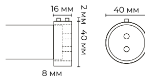
Торцевое крепление для профиля 17x30мм
