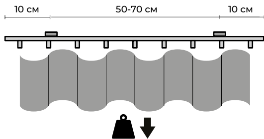
Распределенная нагрузка 2 кг на 1 пог.м карниза
