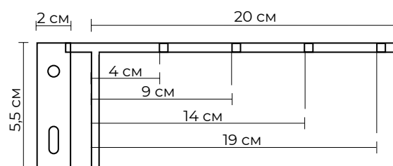
Кронштейн стеновой с крышкой / без крышки 20 см
