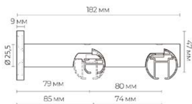
Двухрядный кронштейн
