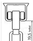
Глайдер роликовый
