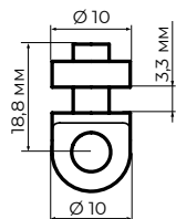
Глайдер стандартный. Шаг: 8 см Цвет: белый / серый / черный Для карнизов: EX.04 / EX.05
