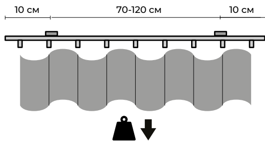
Распределенная нагрузка 3 кг на 1 пог.м карниза
