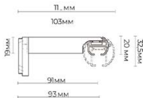
Однорядный держатель 9 см
