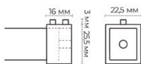
Торцевое крепление для профиля 17x20мм
