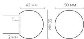
Наконечник Шар Ø35
