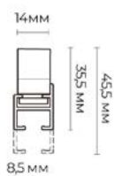
Потолочное парящее крепление 30 мм
