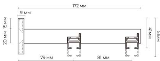
Двухрядный кронштейн
