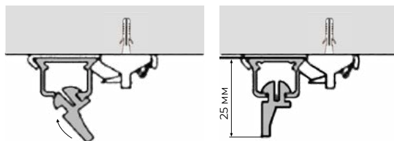
Крепление клик-глайдера
