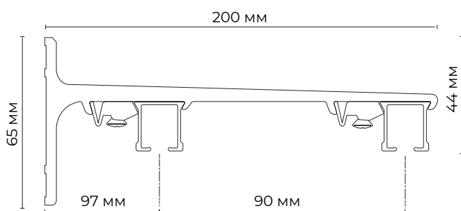
Кронштейн стеновой двухрядный 20 см
