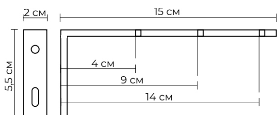
Кронштейн стеновой с крышкой / без крышки 15 см
