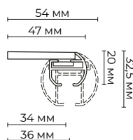
Потолочное с клипсой
