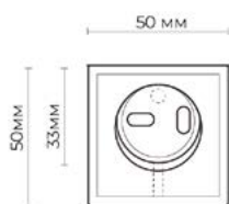
Основа квадратная однорядного кронштейна
