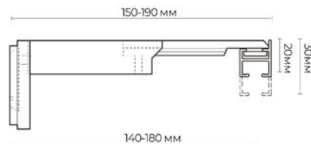
Однорядный телескопический держатель 14-18 см
