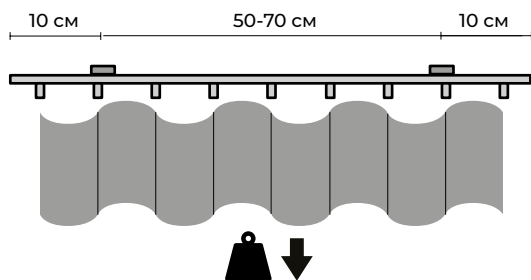
Распределенная нагрузка 2,5 кг на 1 пог.м карниза
