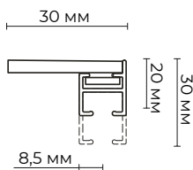
Клипса для поточного крепления 30 мм
