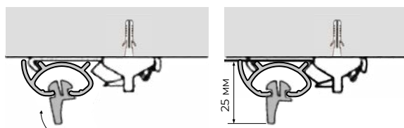
Крепление клик-глайдера
