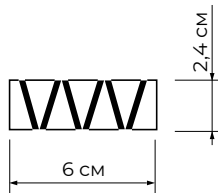
Наконечник Геометрия
