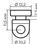
Глайдер широкий. Шаг: 6 см, 8 см Цвет: белый / серый / шампань / черный Для карнизов: EX.06 / DESIGN ROUND / QUADRO
