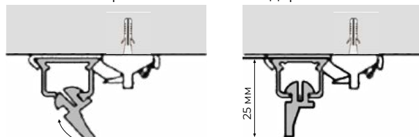
Крепление клик-глайдера
