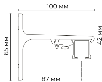
Кронштейн стеновой одnorядный 10 см
