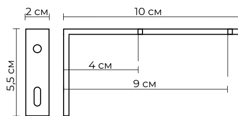
Кронштейн стеновой с крышкой / без крышки 10 см
