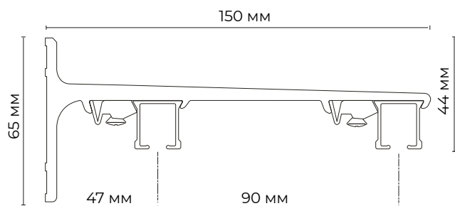
Кронштейн стеновой двухрядный 15 см
