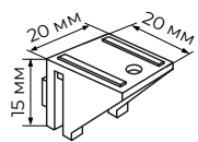
потолочное крепление
