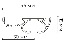
Потолочное крепление
