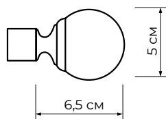
Наконечник Шар классический
