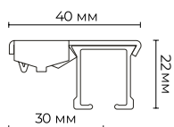
Потолочное крепление
