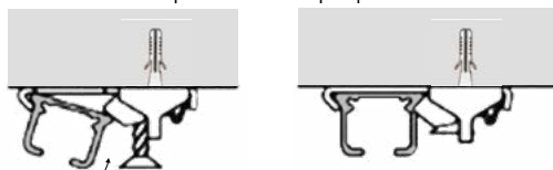
Крепление профиля
