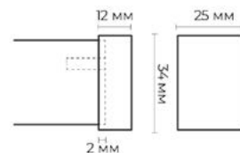
Наконечник Квадро для профиля 17x30 мм
